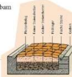
Querschnitt durch die Anlage einer römischen Straße.
